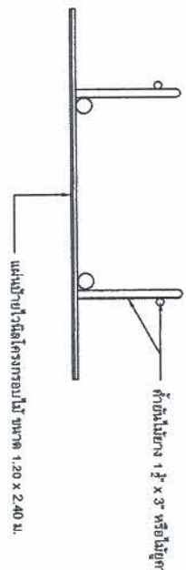
แบบรูปด้านบน 1 : 20
